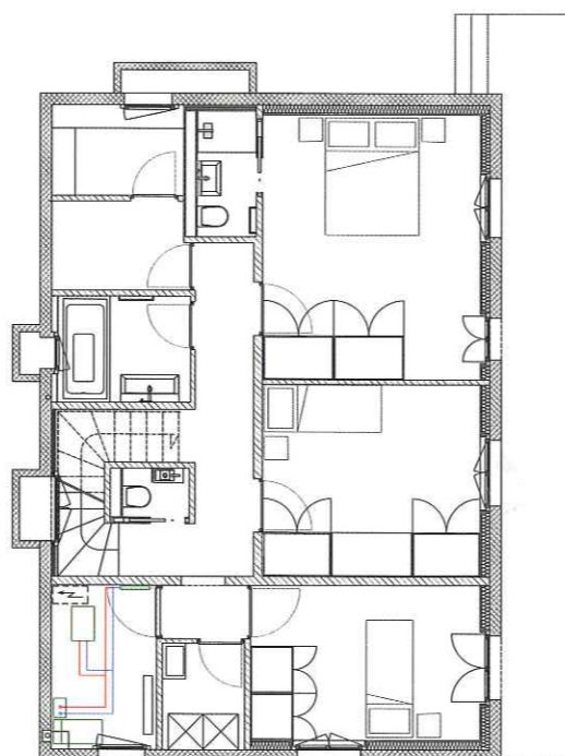
Plan du 1er étage.
